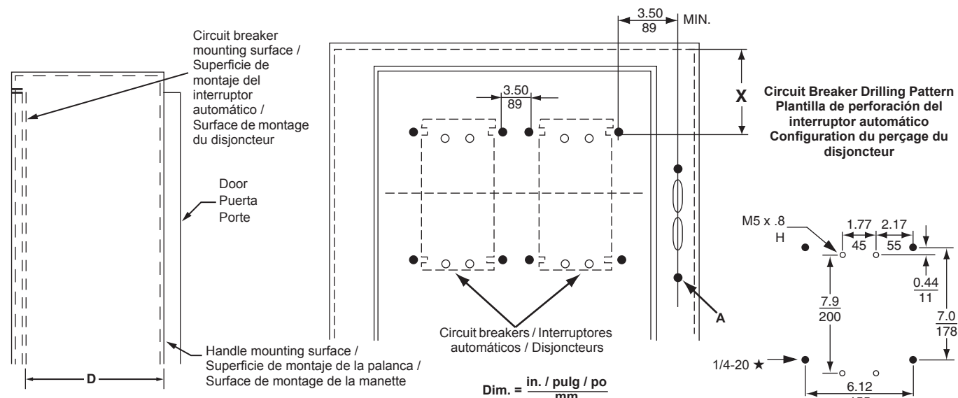
Figure / Figura / Figure 2 : Drilling Dimensions / Dimensiones de perforación / Dimensions de perçage
