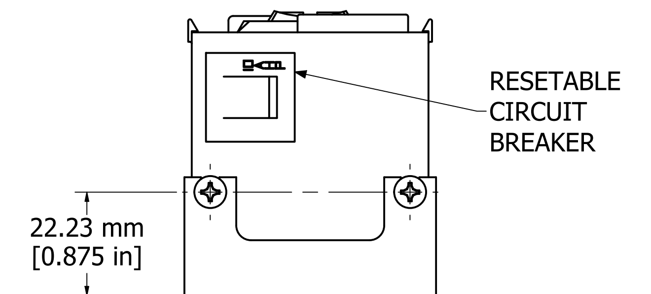
VIEW A-A
