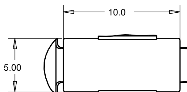
DETAIL A ECHELLE 5:1 SCALE 5:1
