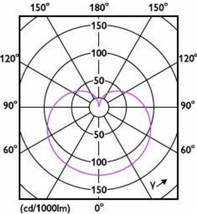
Light Distribution Diagram - 8.8A19/MAS/927-22/FR/P/E26/T20 6/1CT
