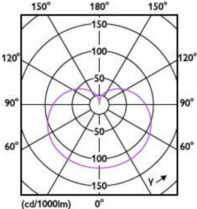
Light Distribution Diagram - 29A21/PER/827/FR/P/E26/WG/HO 4/1PF
