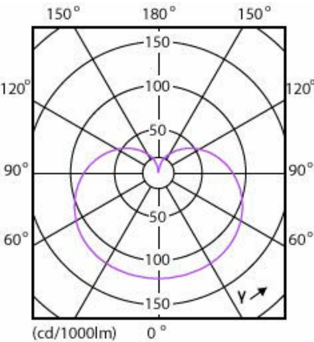
Light Distribution Diagram - 14A19/COR/927/FR/P/E26/DIM/T20 6/1CT
