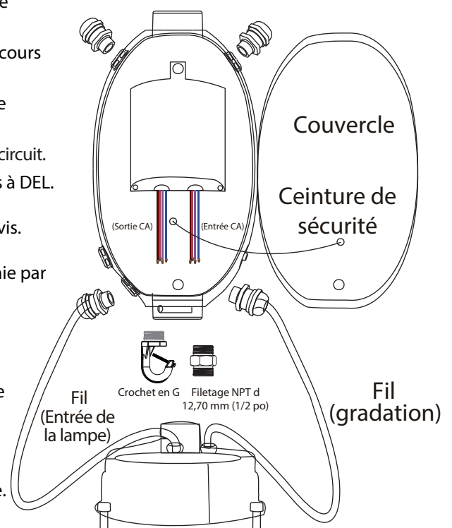
Connecteur étanche
